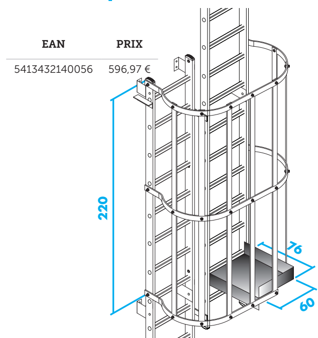
Palier de repos en tôle larmée « brute »
