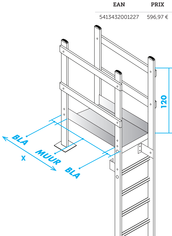
Plateforme de franchissement en tôle larmée « brute » X = 2 \times BLA + \text{ÉPAISSEUR DE MUR}
