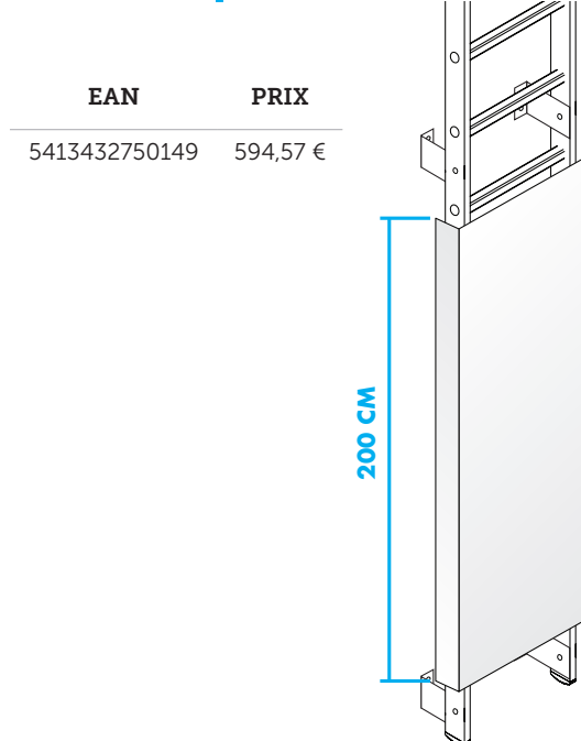
Panneau d'accès en tôle larmée « brute »
